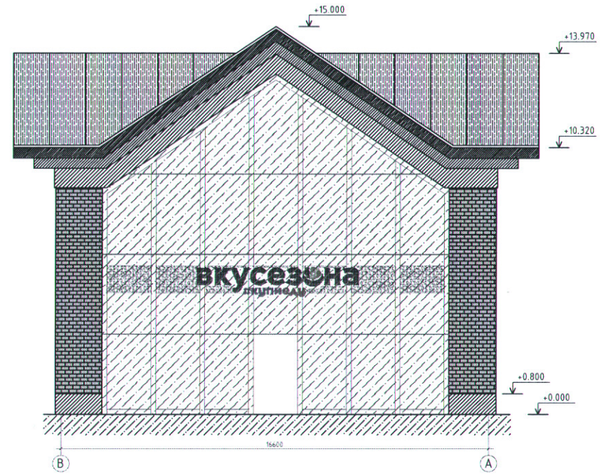
ФАСАД В ОСЯХ В-А
