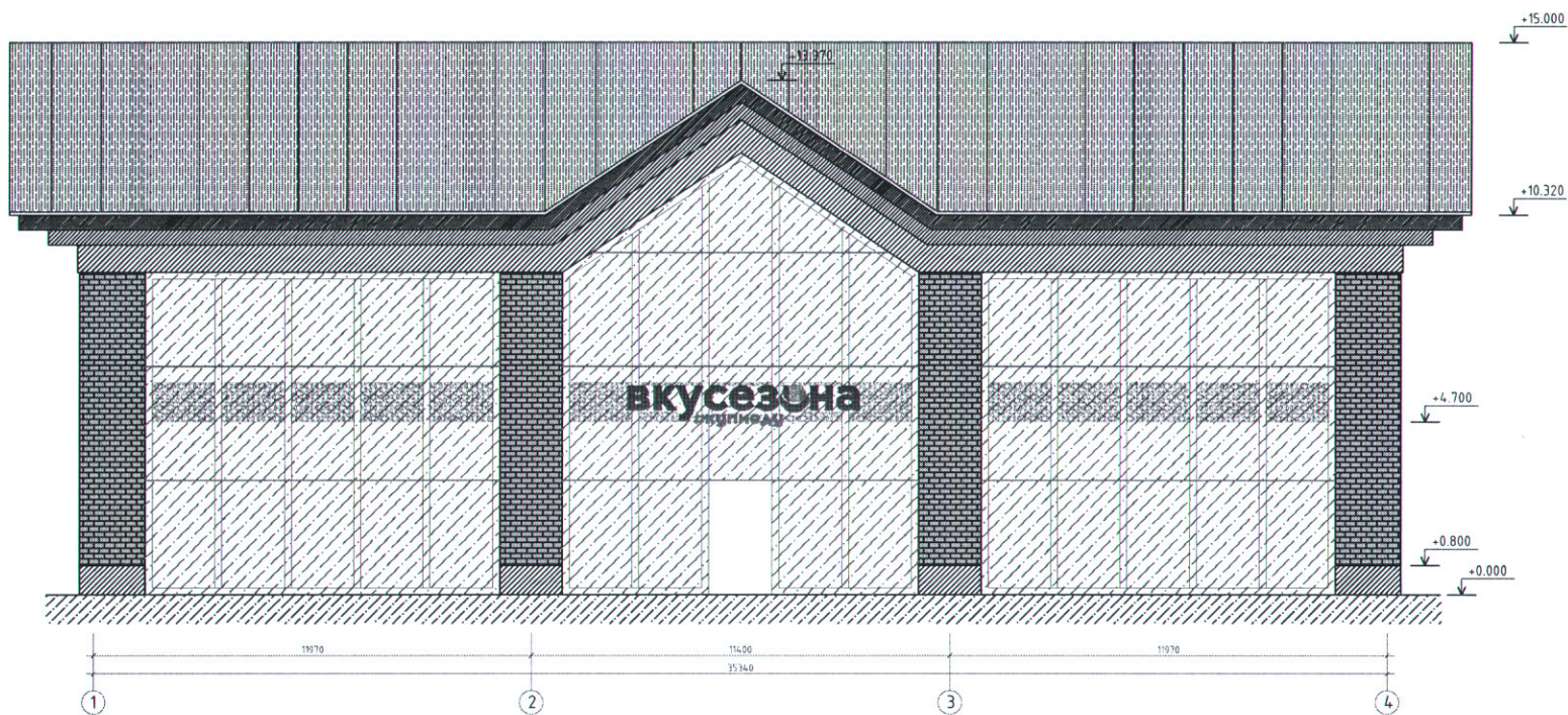
ФАСАД В ОСЯХ 1-4
