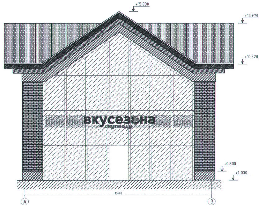
ФАСАД В ОСЯХ А-В
